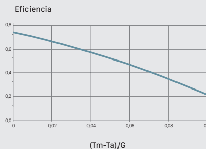
CURVA DE RENDIMIENTO INSTANTANEO
