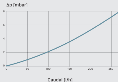
CURVA DE PERDIDA DE CARGA
