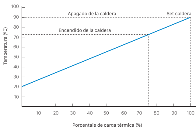
CURVA DE CARGA DEL DEPOSITO DE INERCIA
