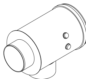
Adaptateur pour tube coaxial Ø100/150 Cod. CGAS000282
