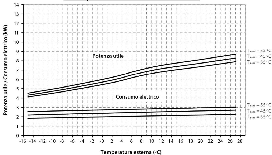
Curve di prestazioni in riscaldamento Dual Clima 9R
