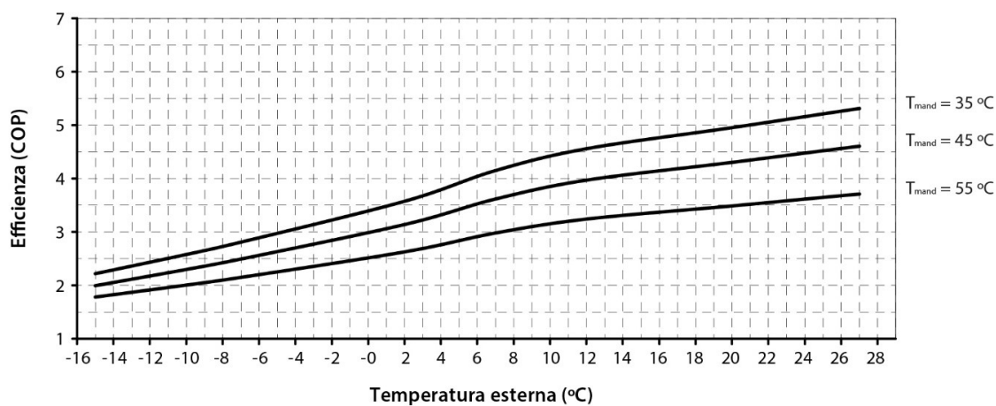
Curve di efficienza in riscaldamento Dual Clima 9R (COP)
