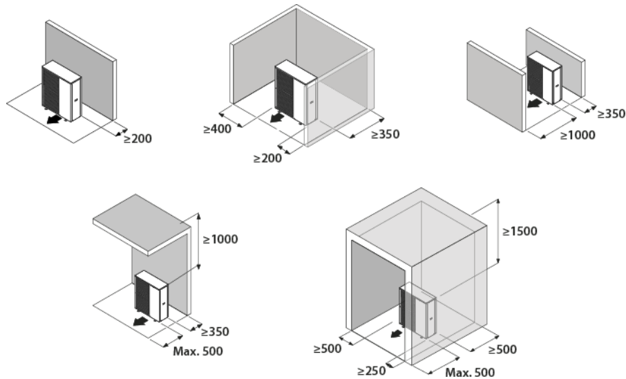
Distancias mínimas para la instalación de una unidad (mm).
