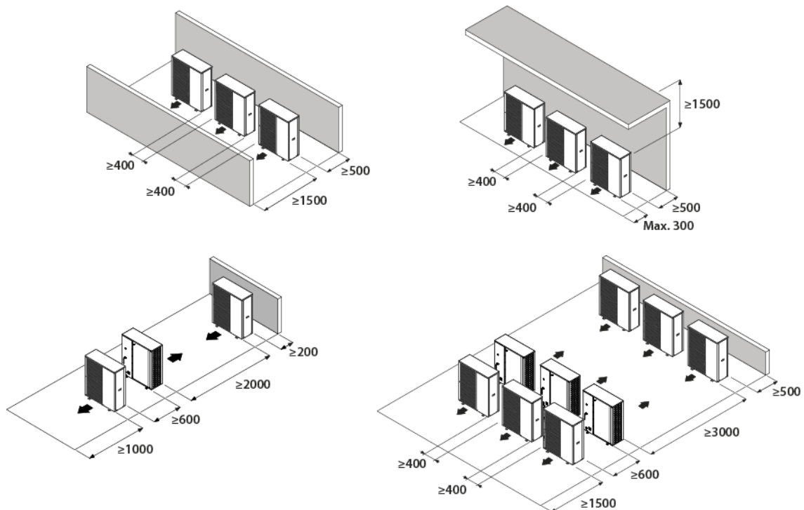
Distancias mínimas para la instalación de múltiples unidades en la misma ubicación (mm).
