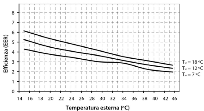
Curve di efficienza in raffreddamento Dual Clima 19R/19RT (EER)
