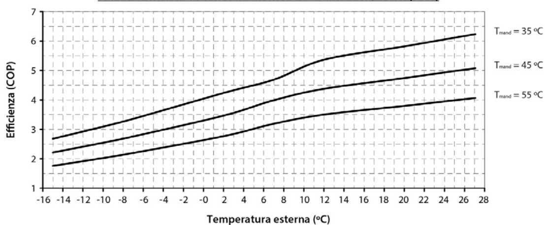
Curve di efficienza in riscaldamento Dual Clima 16R / 16RT (COP)
